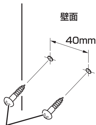
壁掛け用木ネジ×2本(付属品)
